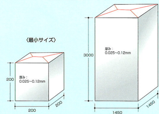
◆パレットカバー寸法図 (mm) ※Xシールの場合
